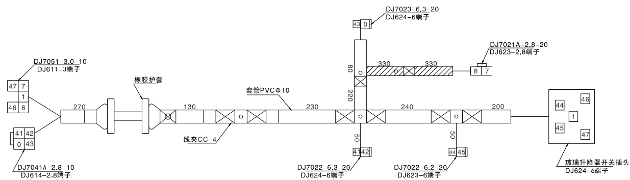
B: HQ6360B-3724330H 后前门线束总成
