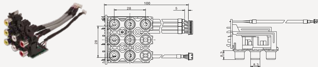
QZ317 11P音响系统插座
