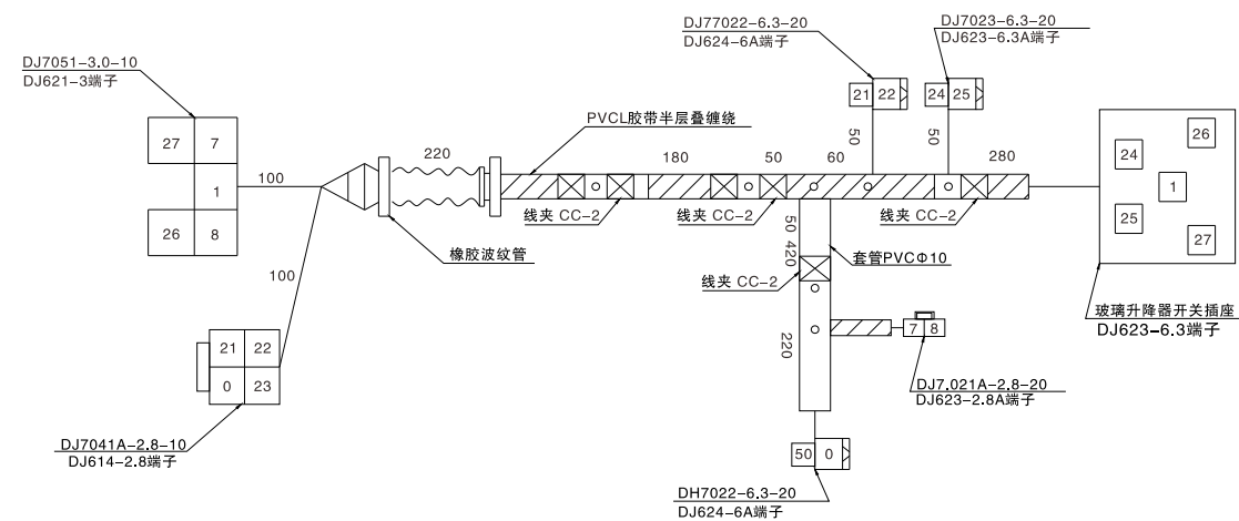
B: HQ6360B-3724330H 后前门线束总成
